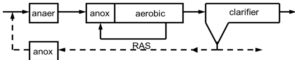
Fig. 14. ISAH-Process
