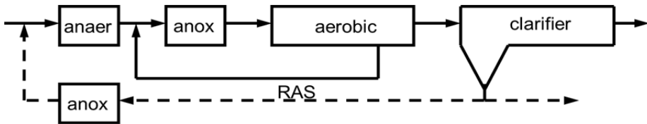
Fig. 10. Johannesburg-Process
