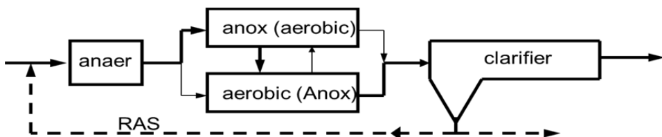
Fig. 12. Biodenipho-Process
